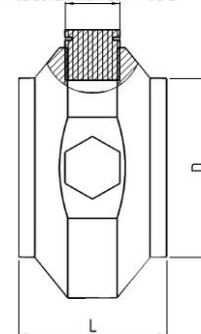
Prise échantillon G3/4" ou G1"
